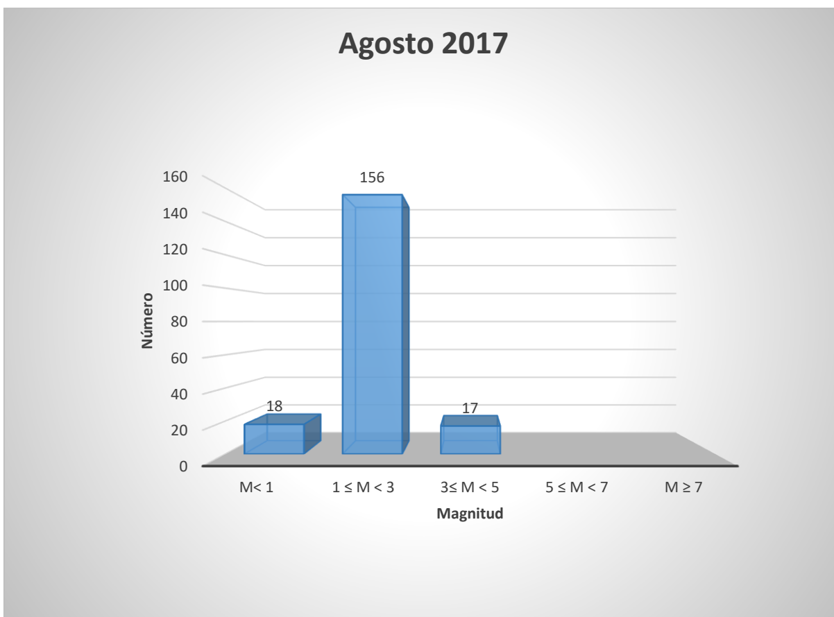
Figura 1. – Gráfica de sismicidad registrada en agosto de 2017.
