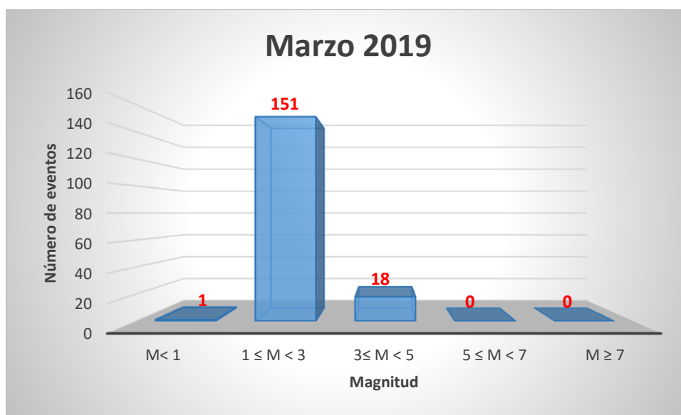
Figura 1. – Gráfica de sismicidad registrada en marzo de 2019.
