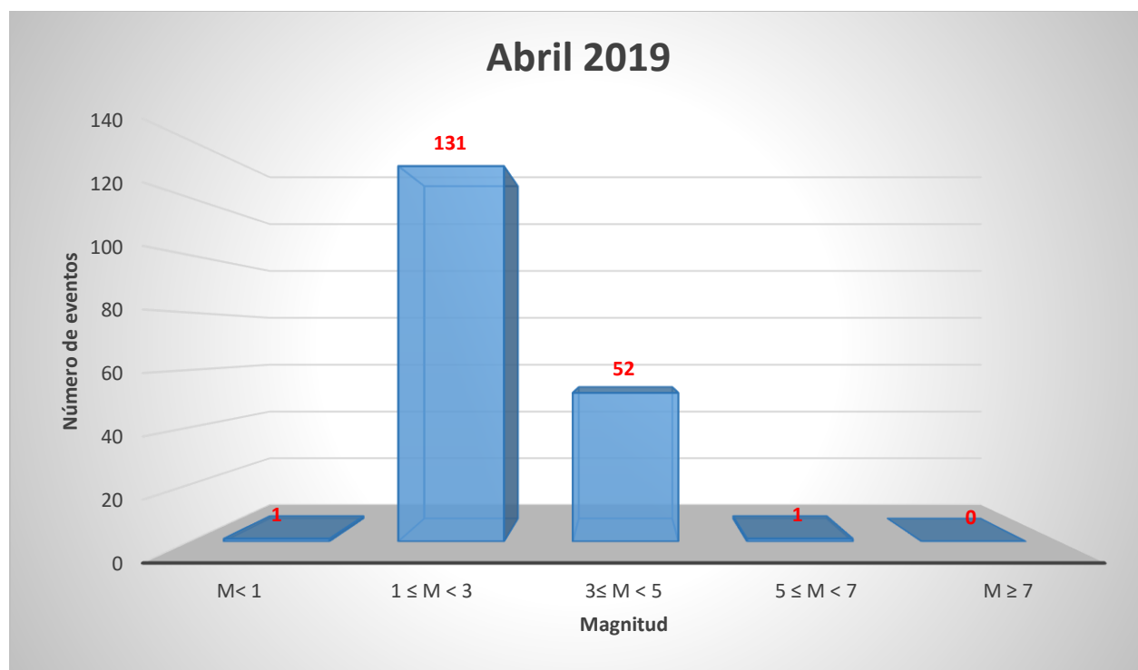
Figura 1. – Gráfica de sismicidad registrada en abril de 2019.
