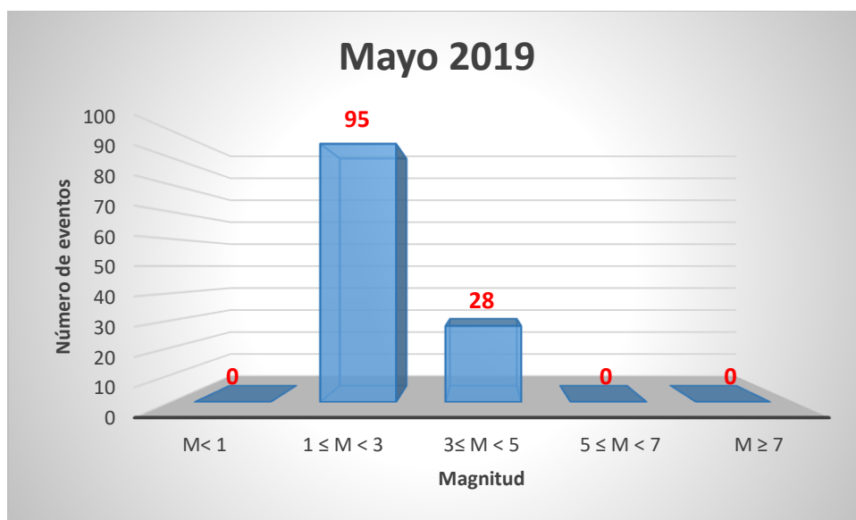
Figura 1. – Gráfica de sismicidad registrada en mayo de 2019.
