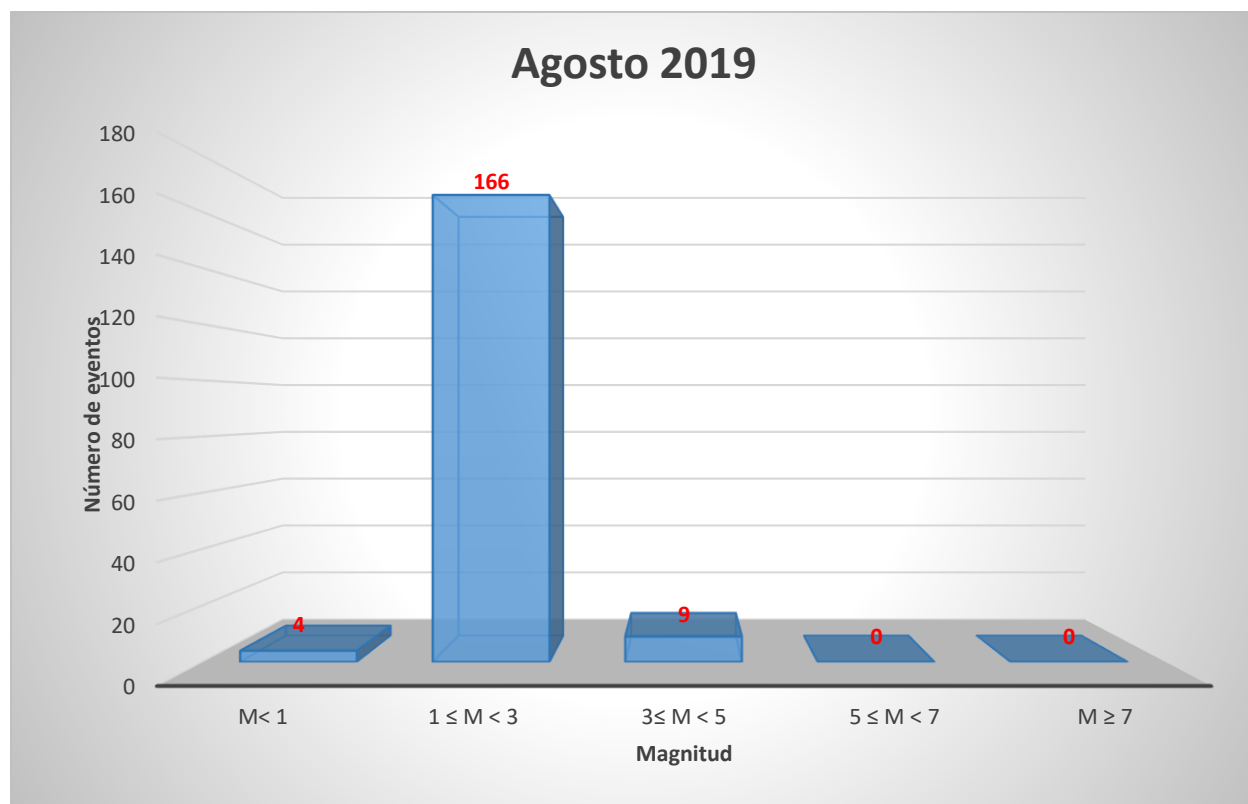
Figura 1. – Gráfica de sismicidad registrada en agosto de 2019.
