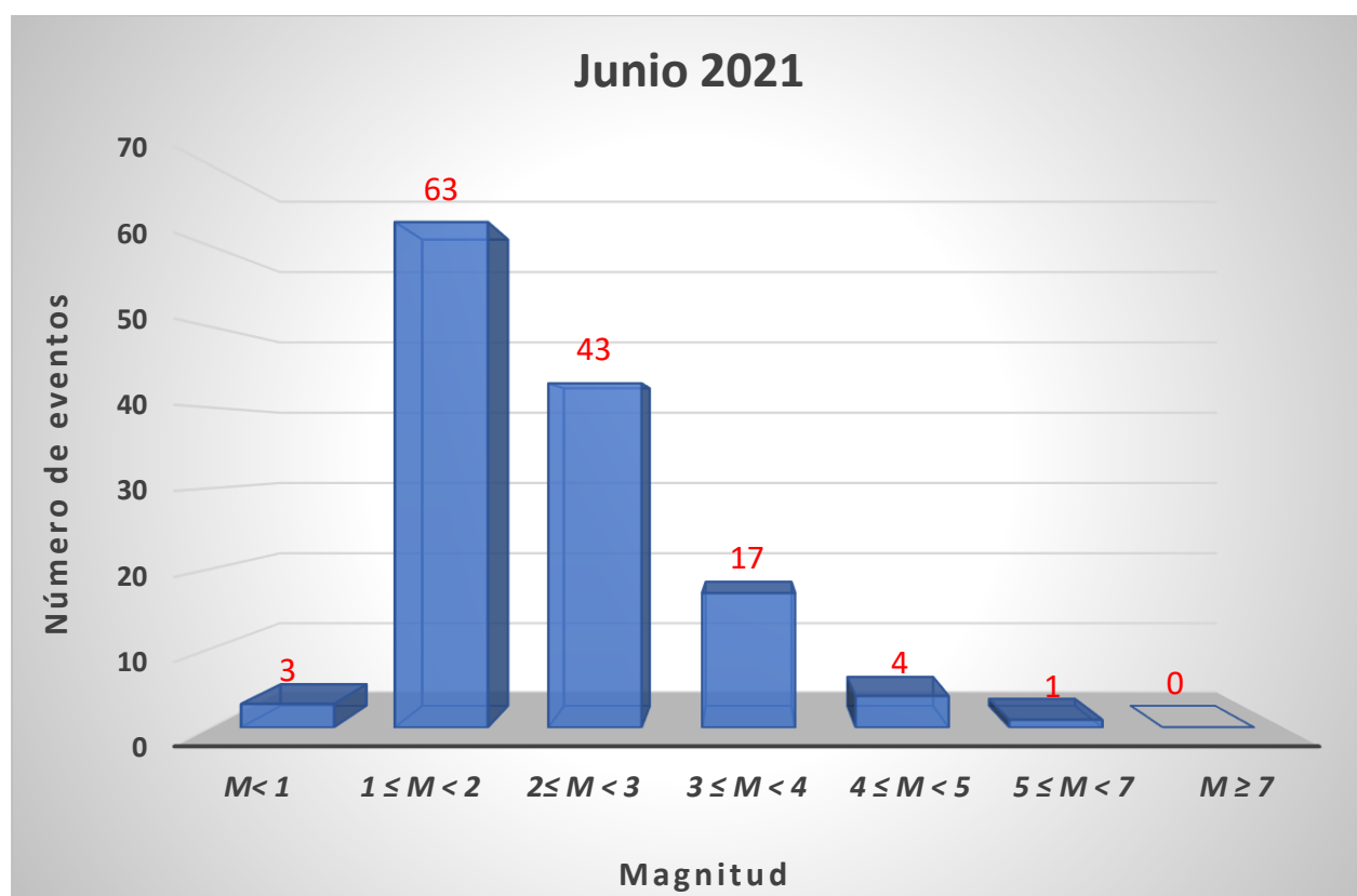
Figura 6.- Gráfico de sismicidad registrada por RSC en junio 2021
