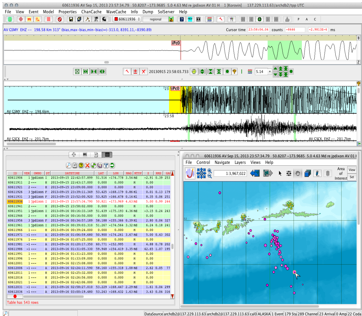
Figura 5.- Interfaz Jiggle
