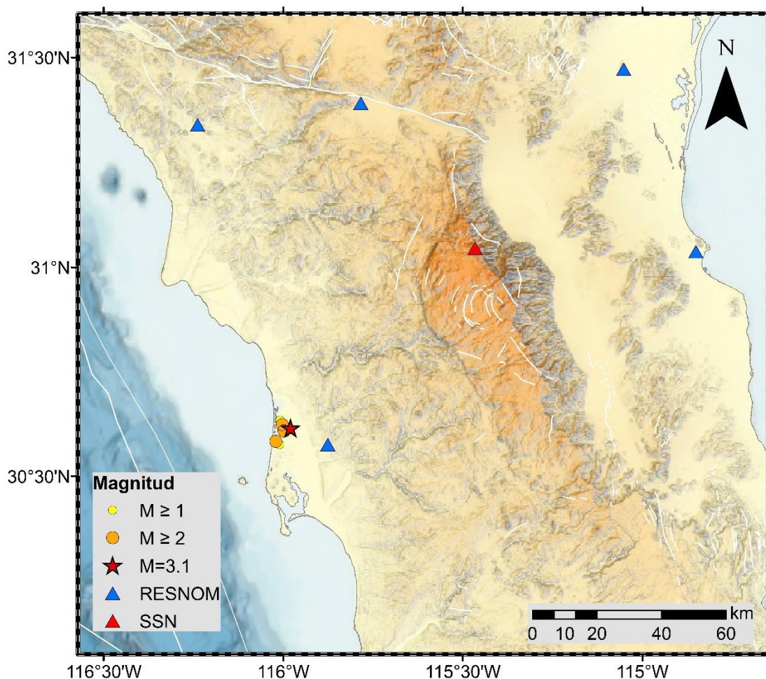
Figura 1. Mapa epicentral del sismo del día 11 de octubre de 2025, magnitud M 3.1, registrado a las 06:29:39 (hora UTC).
