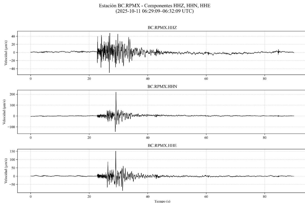
Figura 3. Registros sísmicos del evento principal (M 3.1) de la estación RPMX, de la RESNOM, localizada a 20km del epicentro.
