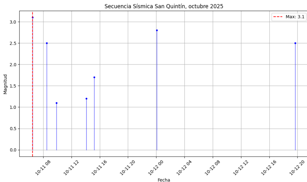
Figura 2. Gráfica de distribución magnitud contra tiempo de la secuencia sísmica del 11 de octubre de 2025, compuesta por 7 sismos localizados en San Quintín, Baja California.
