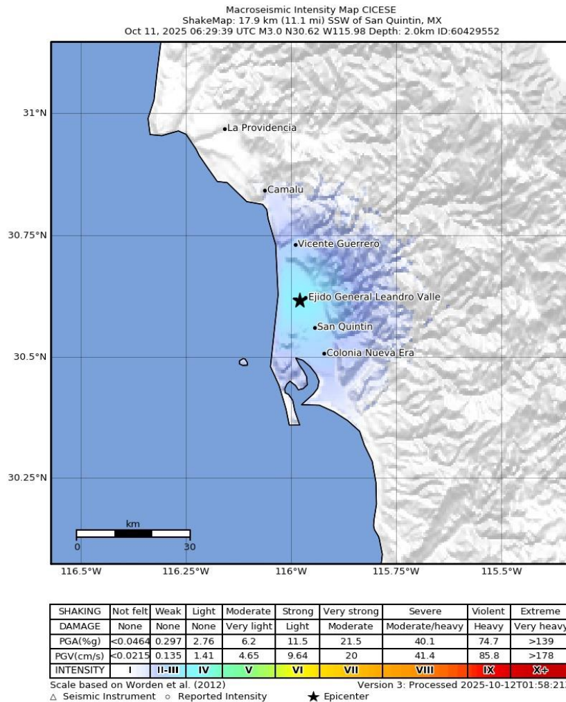
Figura 4. Mapa de intensidades estimadas a partir de aceleraciones registradas durante el sismo del día 11 de octubre de 2025, magnitud M 3.1, registrado a las 06:29:39(hora UTC).
