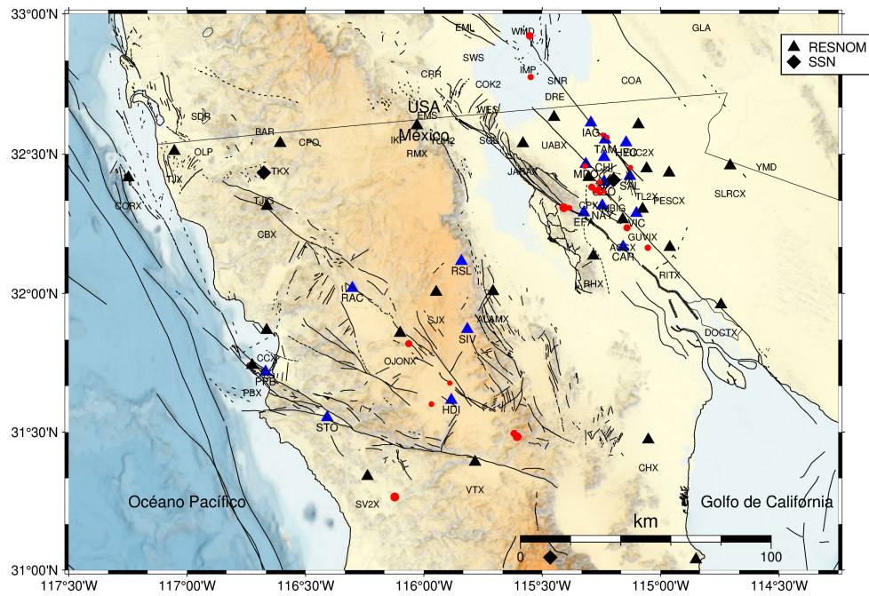
Figura 4: Epicentros (círculos) de sismos registrados por RANOM y localizados en su mayoría, a partir de los datos de las estaciones de RESNOM y de la Red del Sur de California. Las estaciones de RANOM están representadas por triángulos, en tanto que las estaciones de RESNOM y de la Red del Sur de California, se encuentran representadas por pentágonos y cuadros respectivamente.
